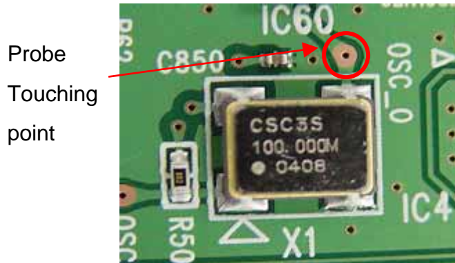
OSC(X1)
